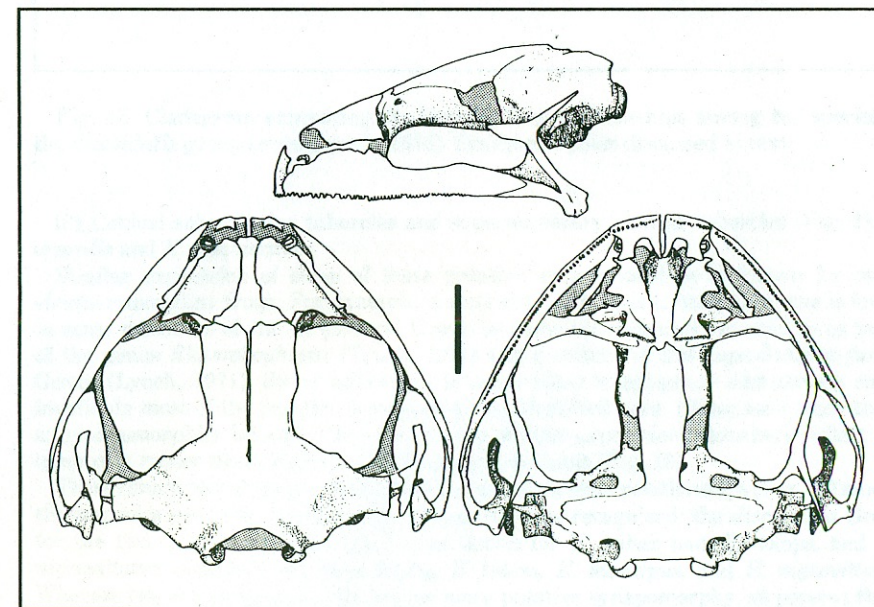
Fig. 11. Cranium of Eleutherodactylus nigrovittatus , USNM 222807. Scale equals 2 mm.
